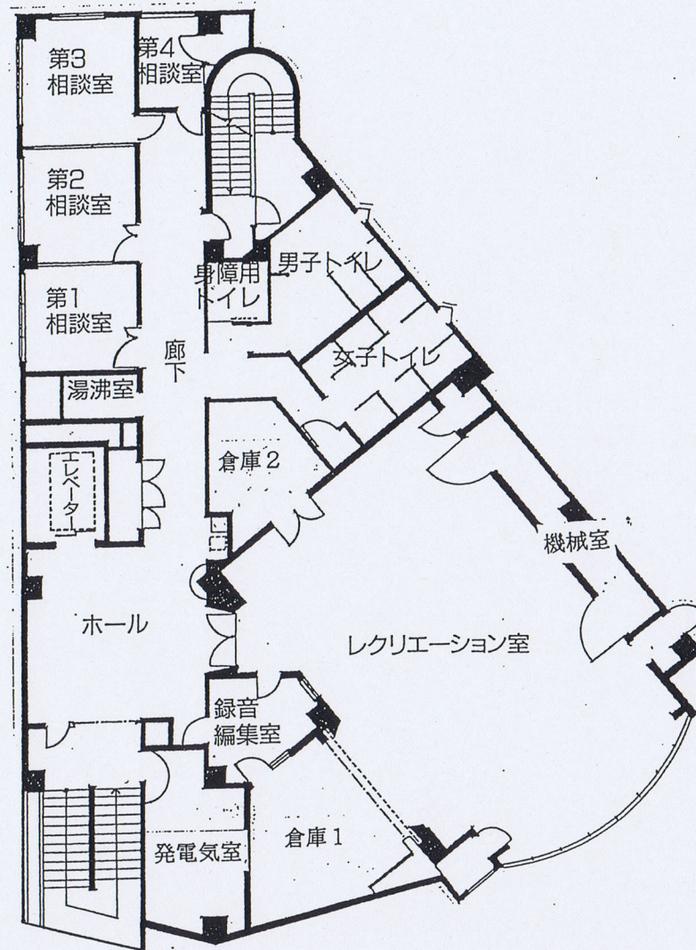
2階平面図
