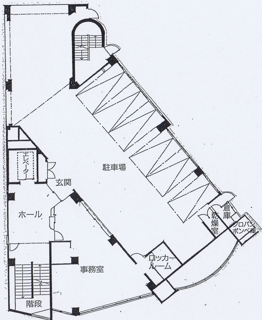
1階平面図
