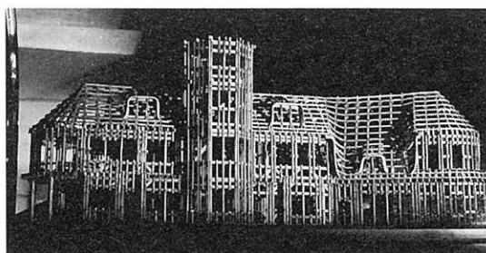
城山荘（三井大磯別邸）軸組模型（当館蔵）
