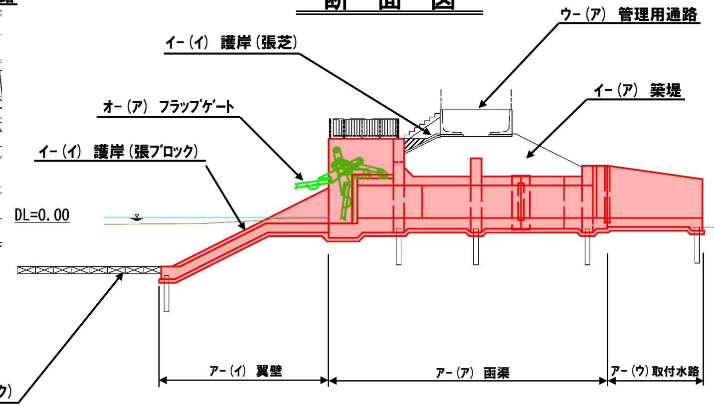
断面図
