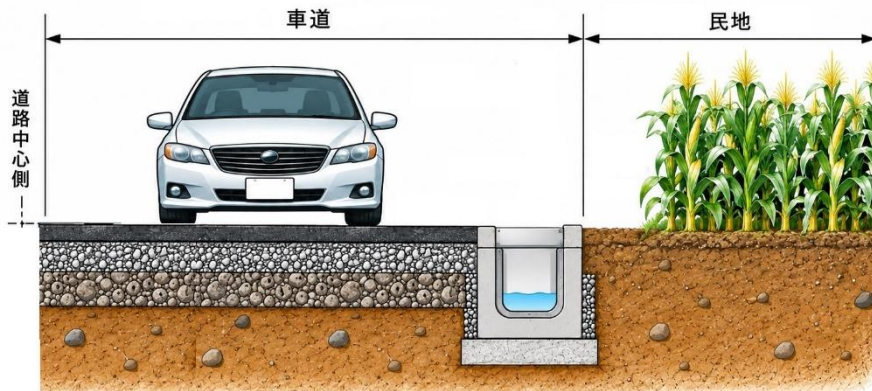
横断図（現況）
