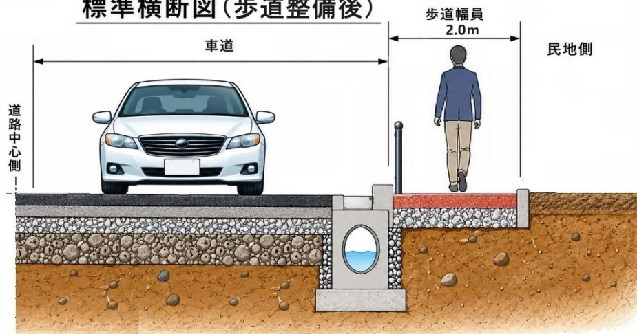
標準横断図（歩道整備後）
