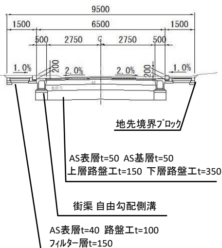
幹線21号線 標準横断面図
