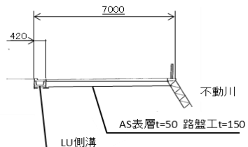
生沢月京1号線 標準断面図
