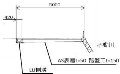
生沢月京1号線 標準断面図
