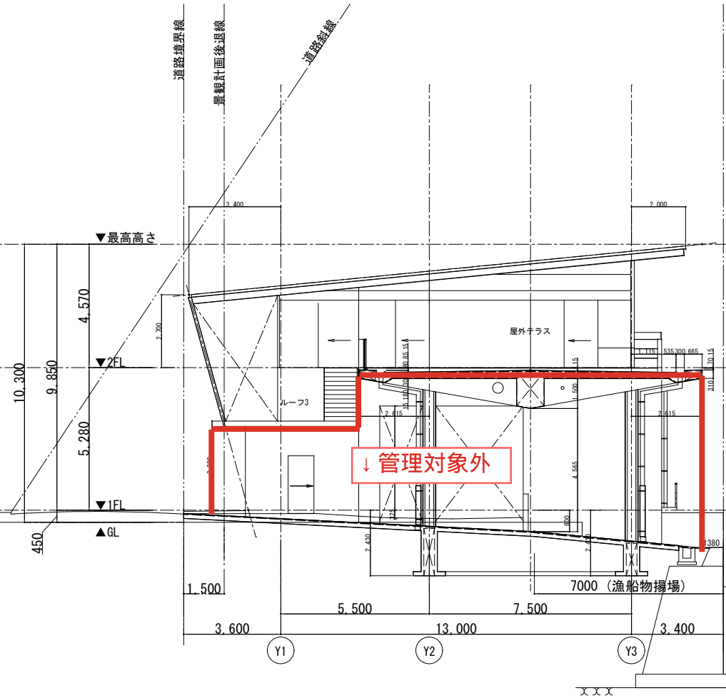
断面図 2
