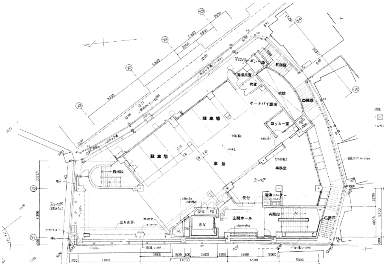
1階平面図
