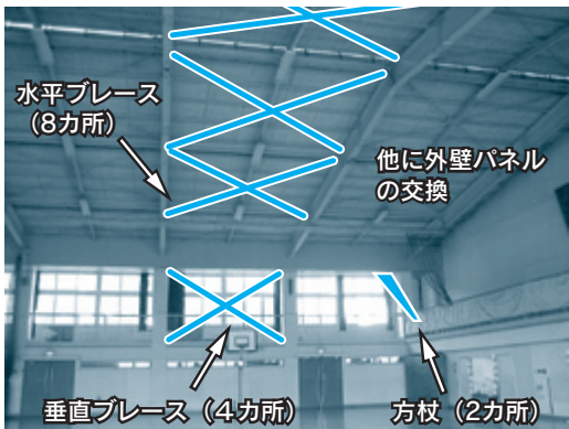
補強が必要な体育館の屋根
