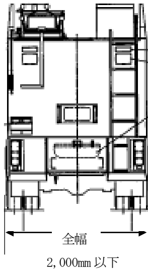
【後面】
