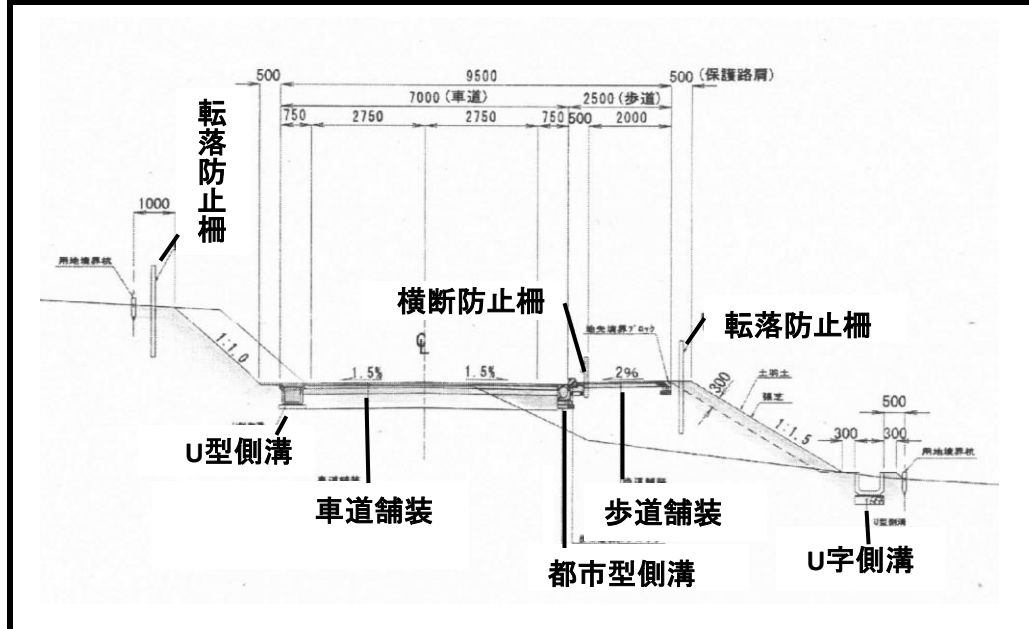
標準構造図等
