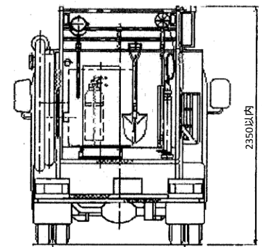
后面图
