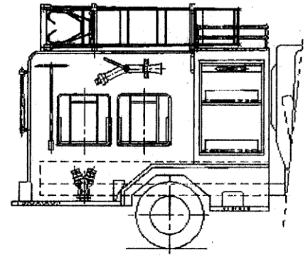
右侧面图
