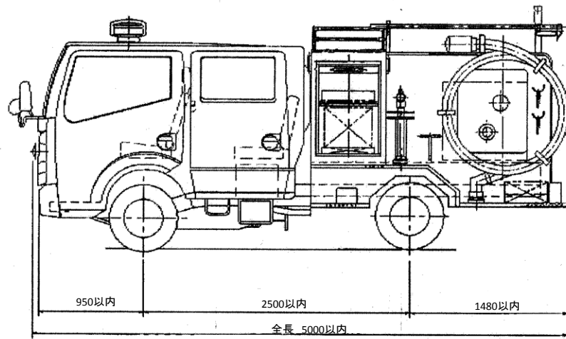
左侧面图
