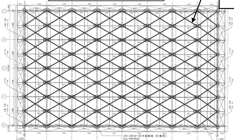
天井伏面 補強ブレース配置図
