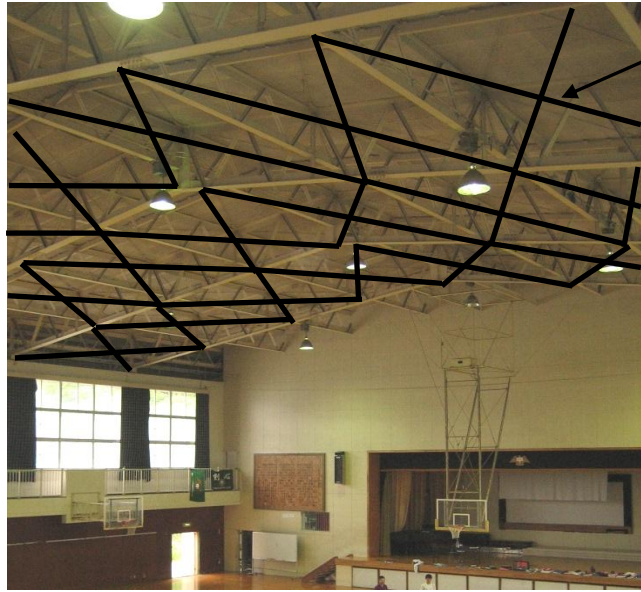
天井伏面 補強ブレース配置図
