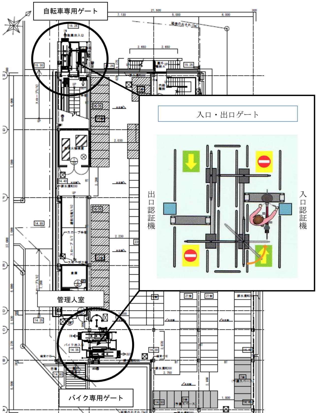
自転車等駐車場配置図（地下1階平面図）
