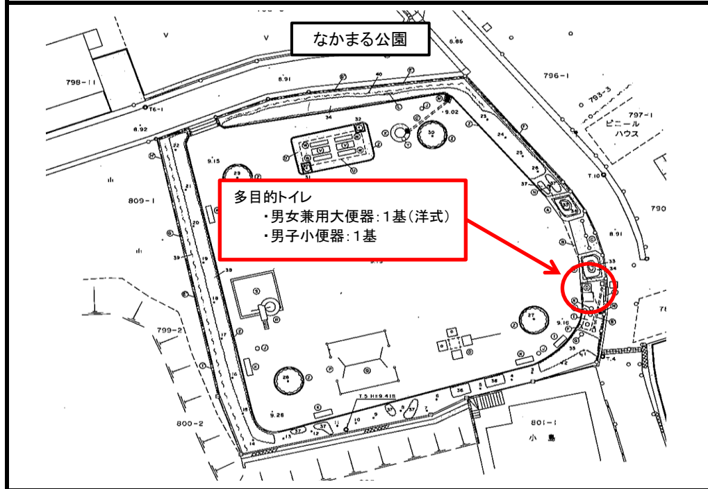
計画平面図
