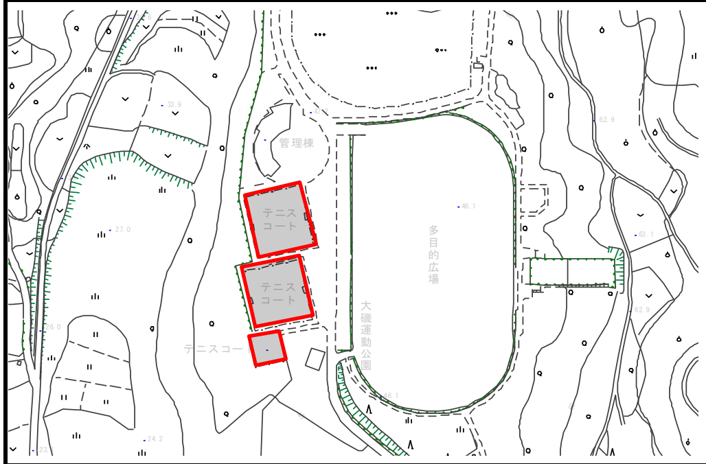
計画平面図
