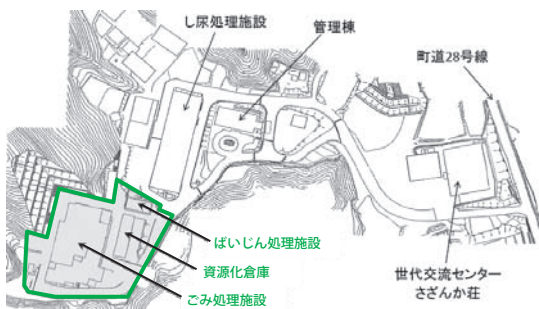
大磯町美化センター施設配置図
