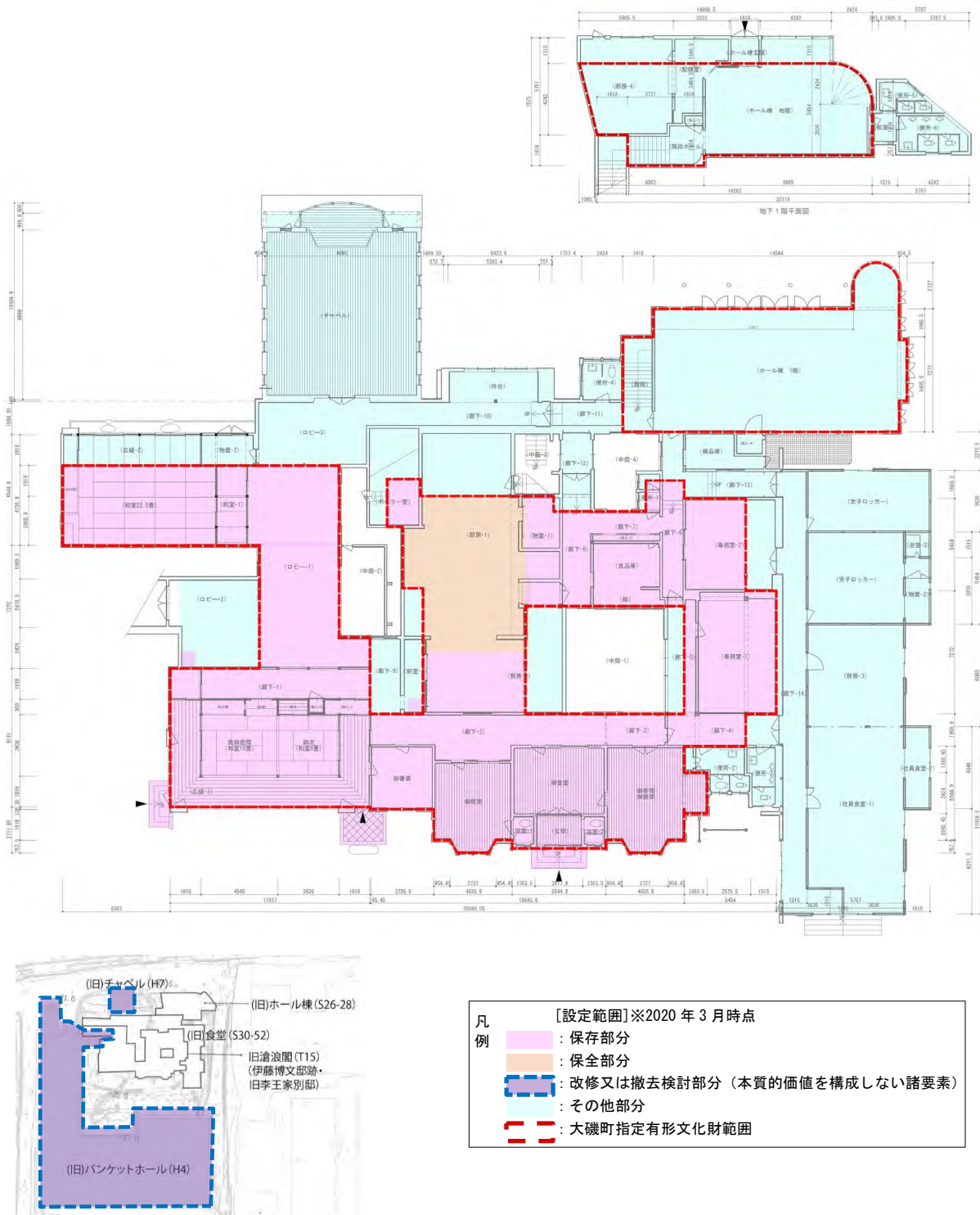
図 28 旧滄浪閣（伊藤博文邸跡・旧李王家別邸）部分の設定（平面）
