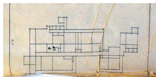
図 13 旧大磯町行政資料 古河虎之助昭和5年届出図面(部分) (水沼淑子.学術講演梗概集 日本建築学会 『旧大隈重信大磯別荘の履歴』2015)
