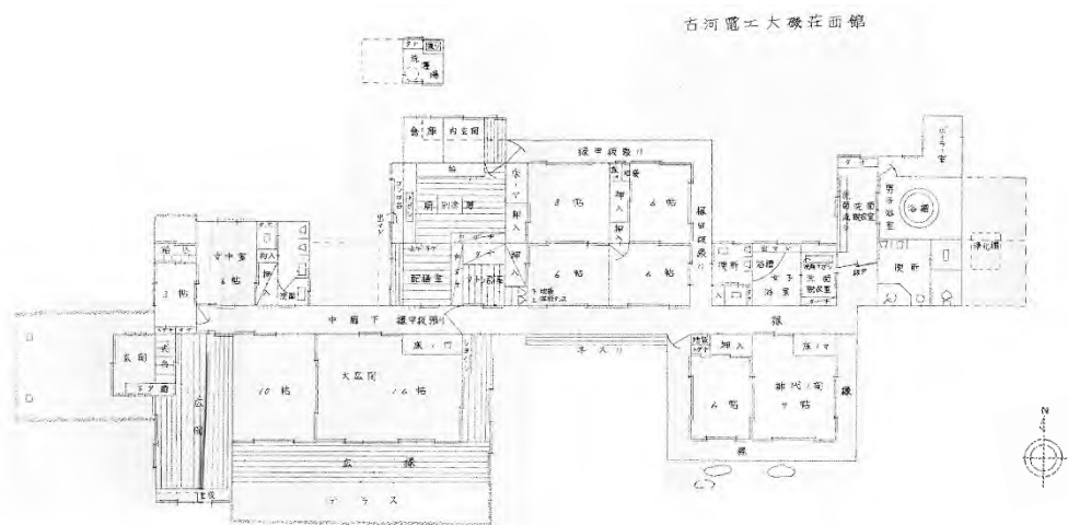
図 14 古河電工大磯荘西館平面図（昭和 34 年以前）
