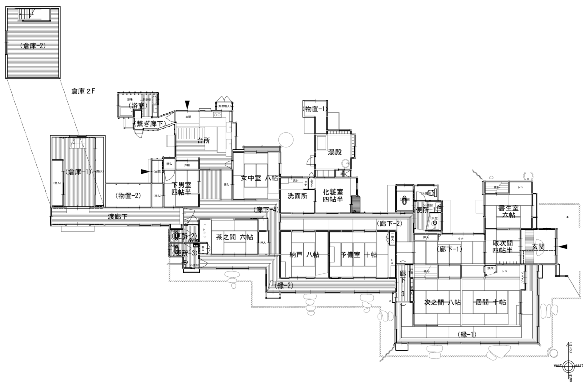
図 21 陸奥宗光別邸跡・旧古河別邸 平面図
