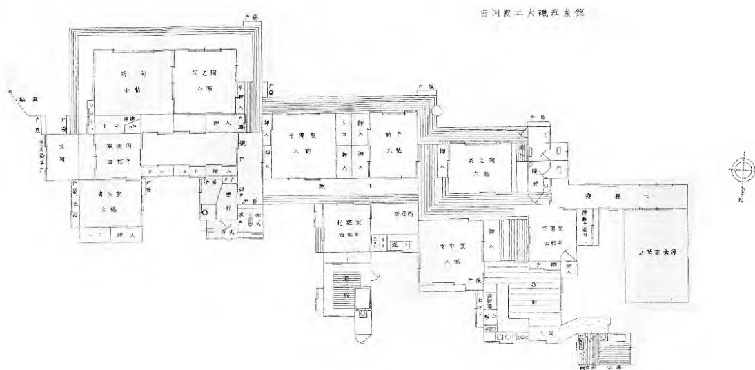
図 19 古河電工大磯荘東館平面図（昭和 34 年以前）
