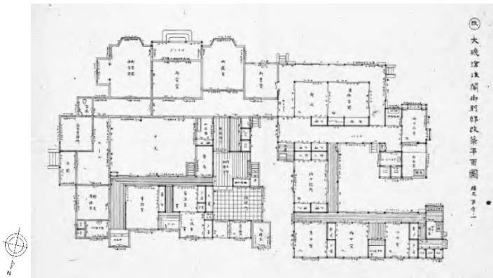
図6 大磯滄浪閣御別邸改築平面図 (東京都立中央図書館特別文庫蔵)
