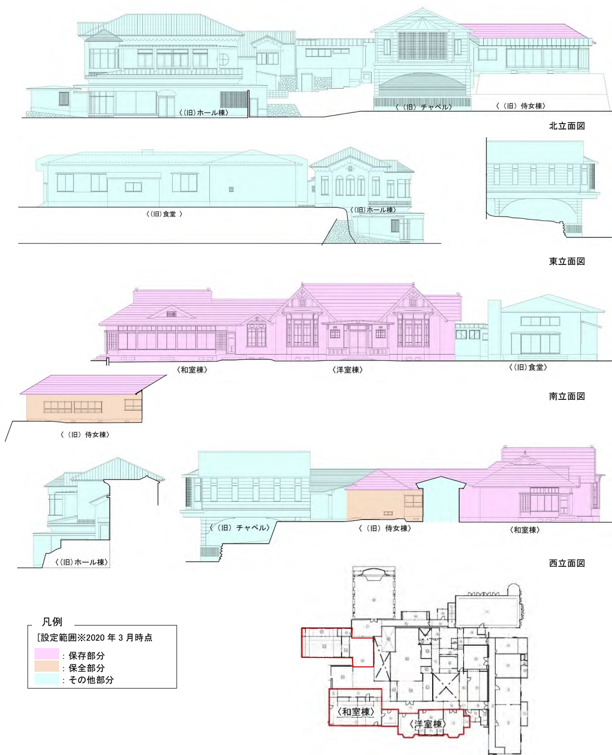
図 29 旧滄浪閣（伊藤博文邸跡・旧李王家別邸）部分の設定（立面）
