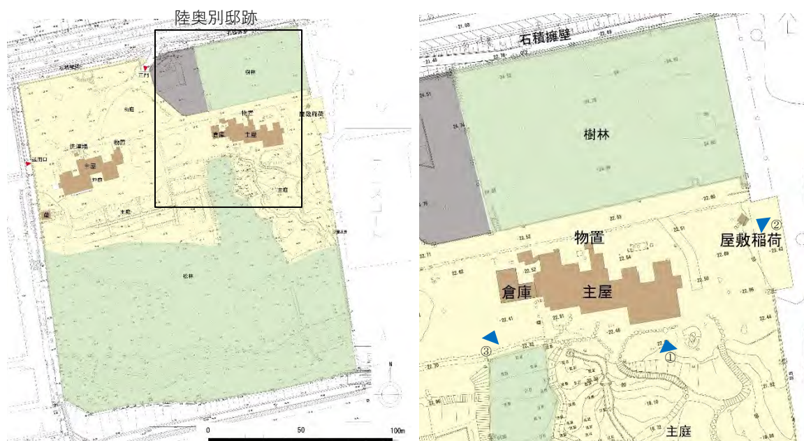
図 20 陸奥宗光別邸跡・旧古河別邸 配置図
