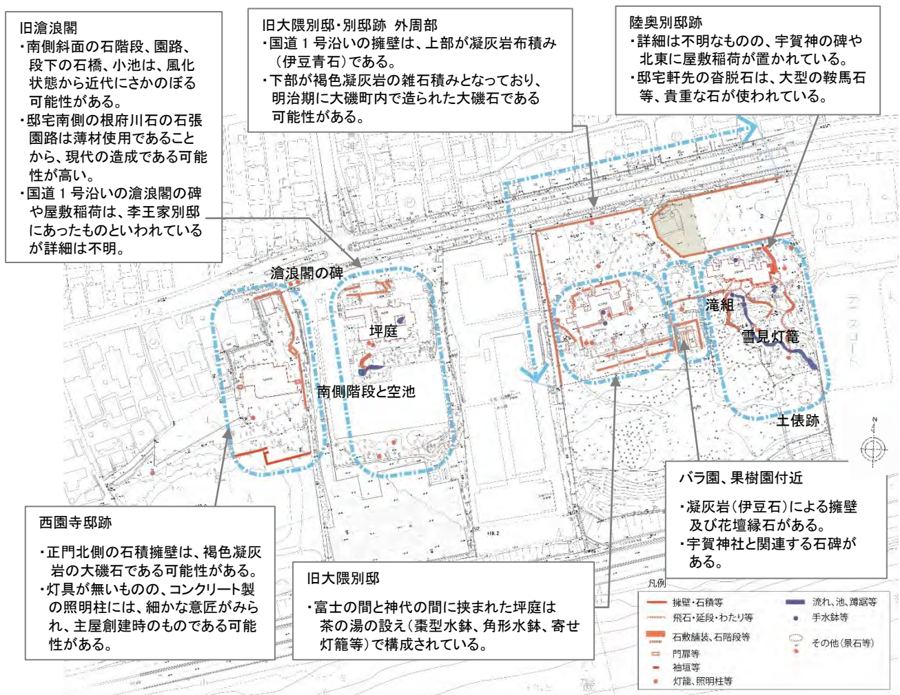
図 38 主な構造物
