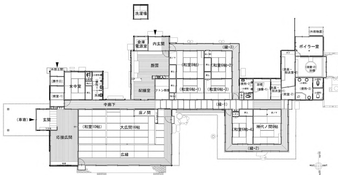
図 16 旧大隈重信別邸・旧古河別邸 平面図
