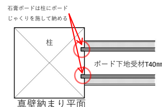
写真44 石膏ボードを用いた壁工法
